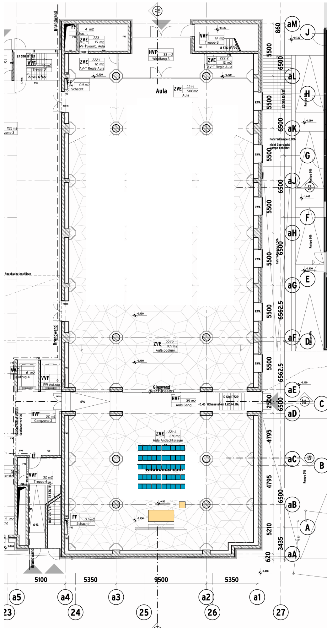
Grundriss EG – B1_Kleine Andacht 50 Personen
