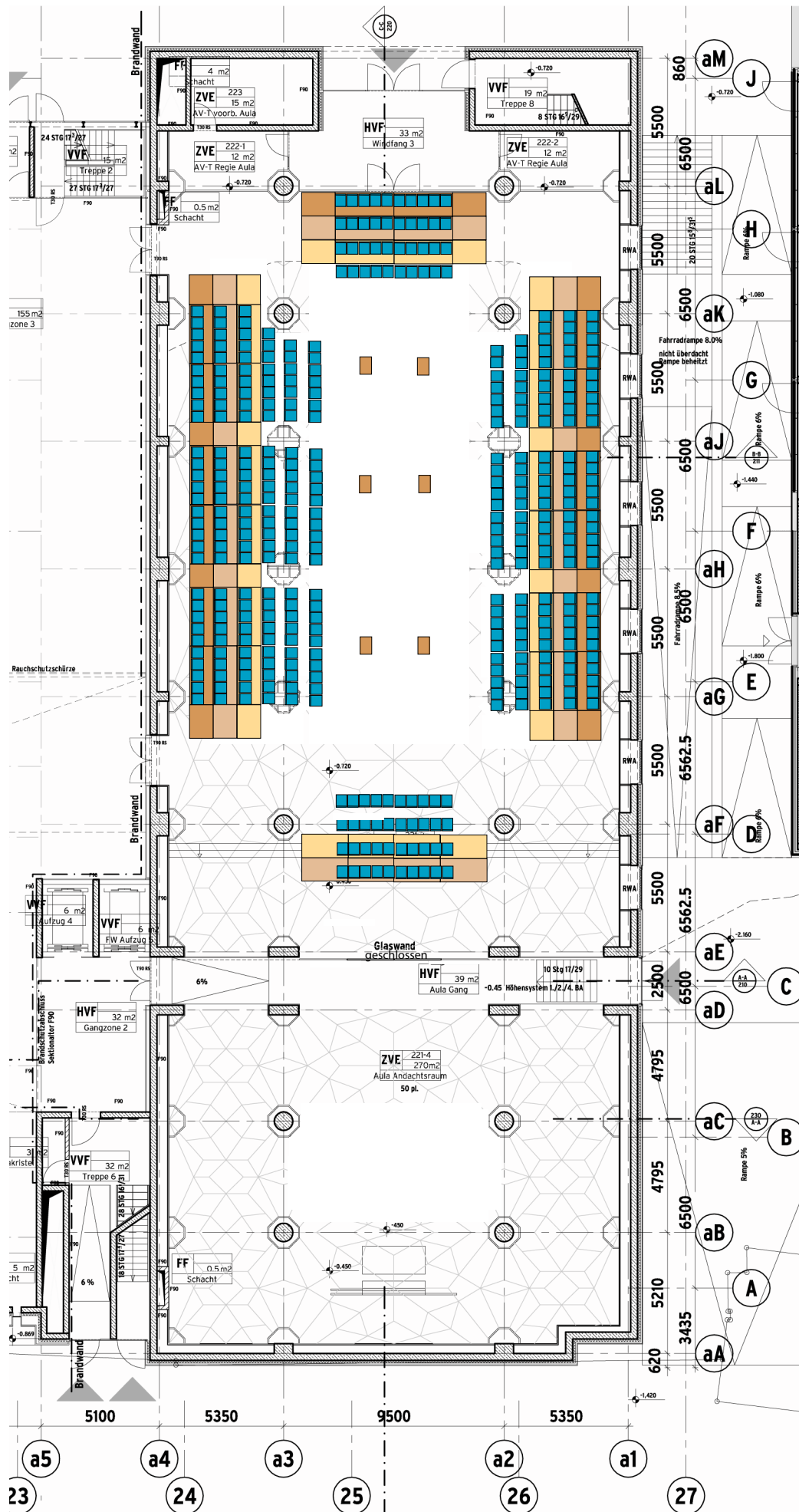
Grundriss EG – E_Wissenschaftl. Disput 374 Personen, max. 550
