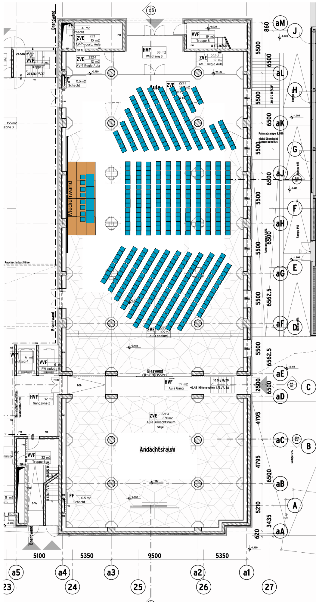
Grundriss EG – F_Festkolloquium 477 Personen, max. 550
